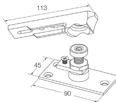
GGHPD16 Bottom Pivot
