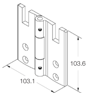
SLF400HN100 Hinge (DRM100)
