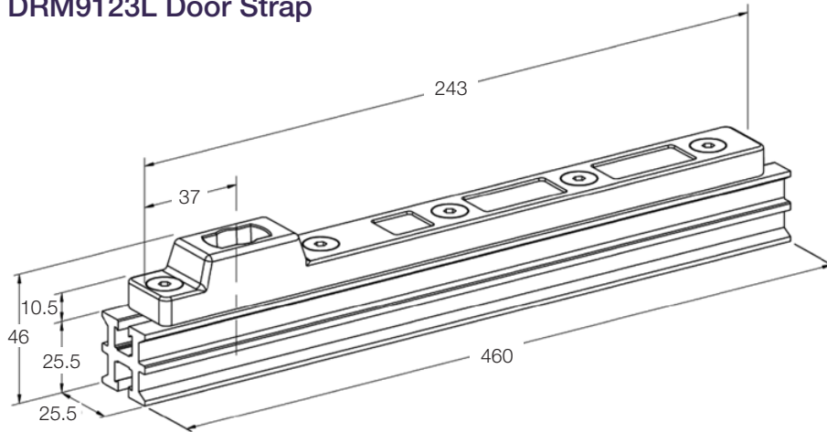
DRM9123L Door Strap
