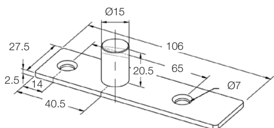
DRMPD24NS15 Top Pivot
