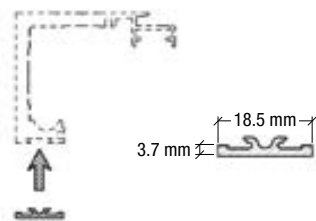
5 GSD52EC End Cap
