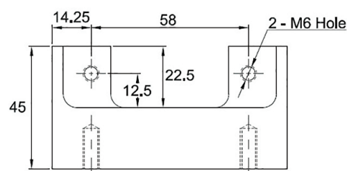
DRM2015 Side Load Top Pivot Block
